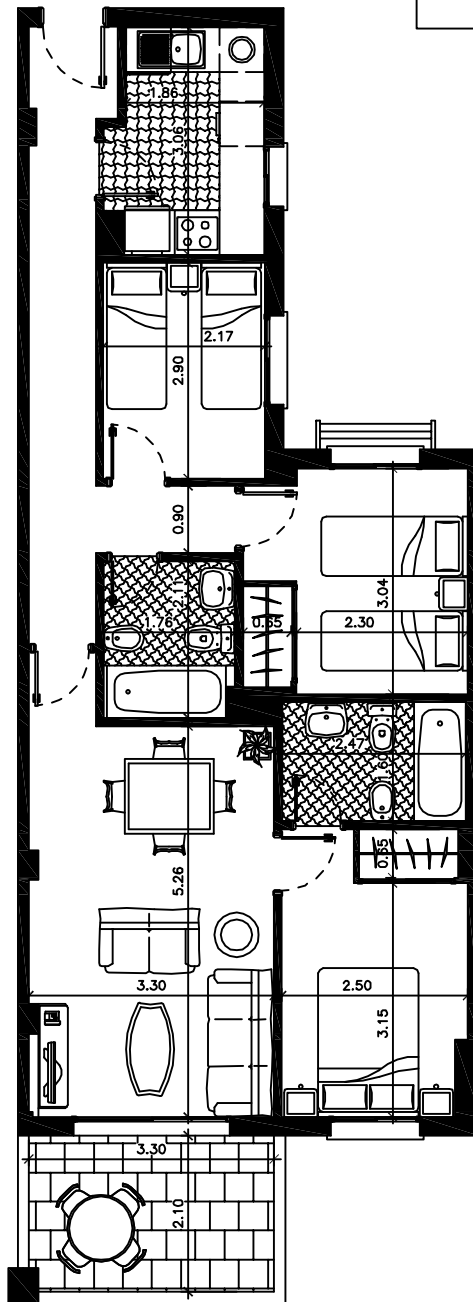
VIVIENDA TIPO D, F Nivel 1, 2 y 3 (Portal 1)
