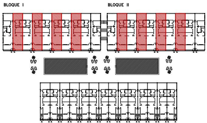
PLANTA GENERAL
